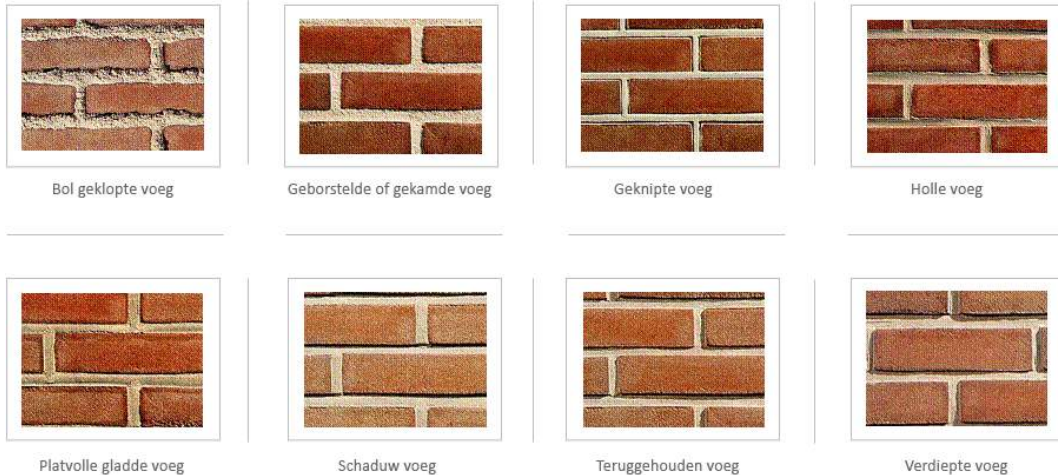
Voorbeelden en technische benamingen van voegwerk
